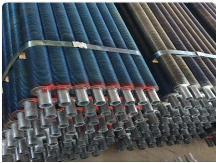
高频焊螺旋翅片管
